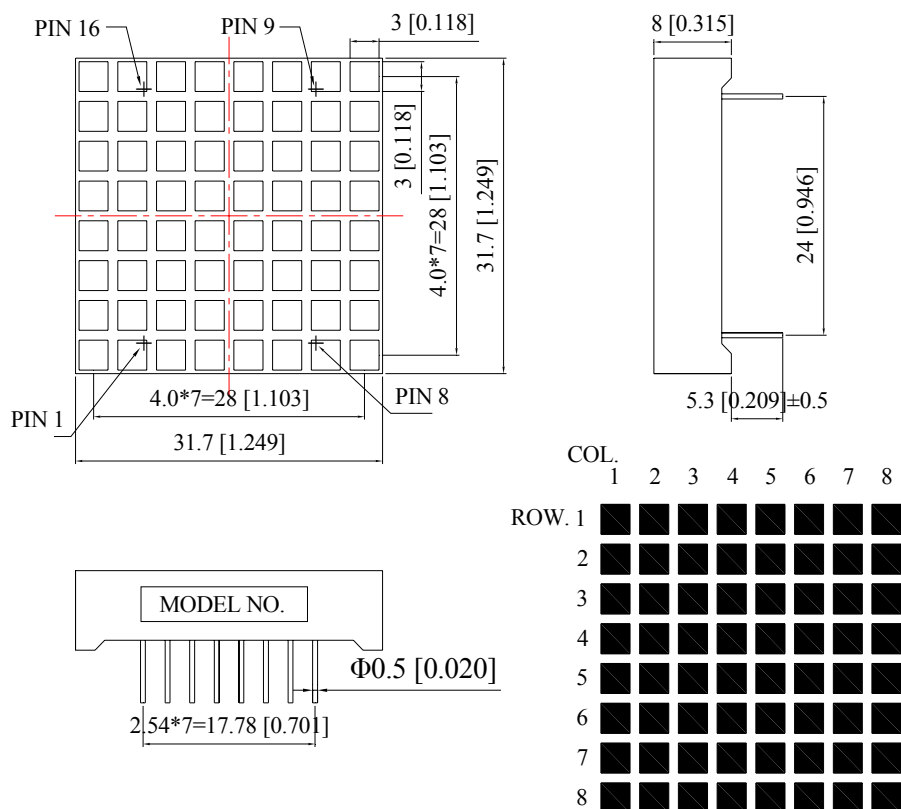
KWM-R30882AVB
