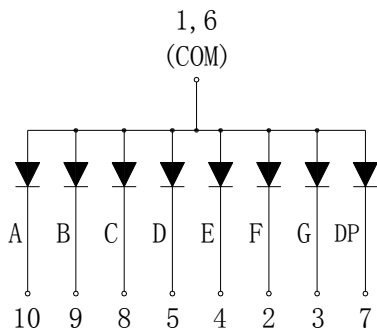
KW1-361AGB
