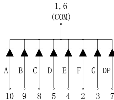
KW1-361CGB
