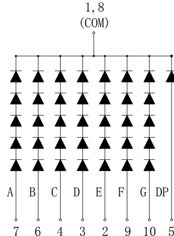
KW1-4001CPGB
