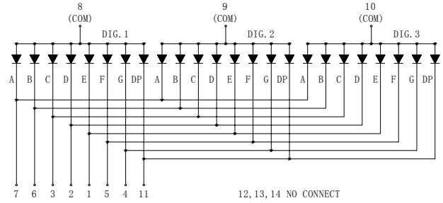
KW3-563ASB
