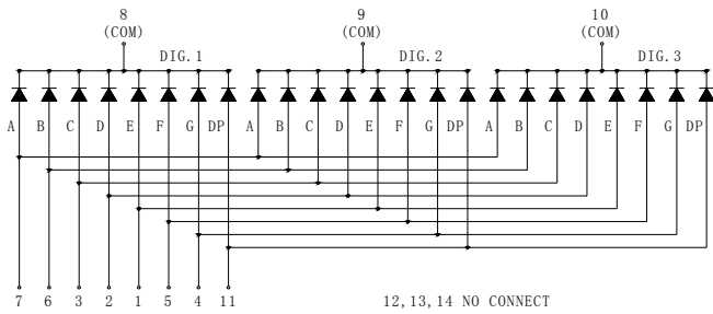
KW3-563CSB
